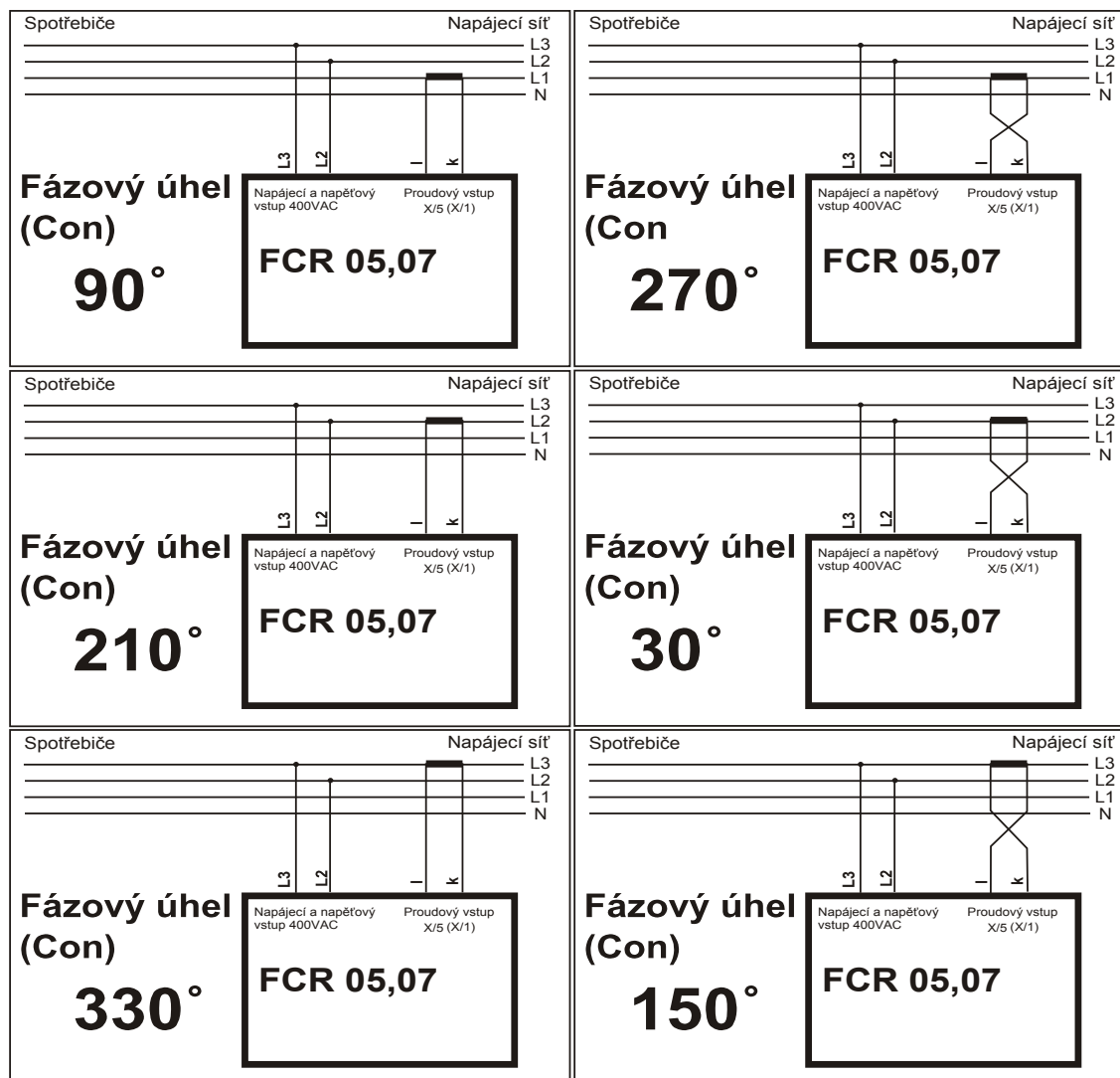
Obr. 4. Nastavení fázového posuvu pro napájecí a měřící napětí 400V
