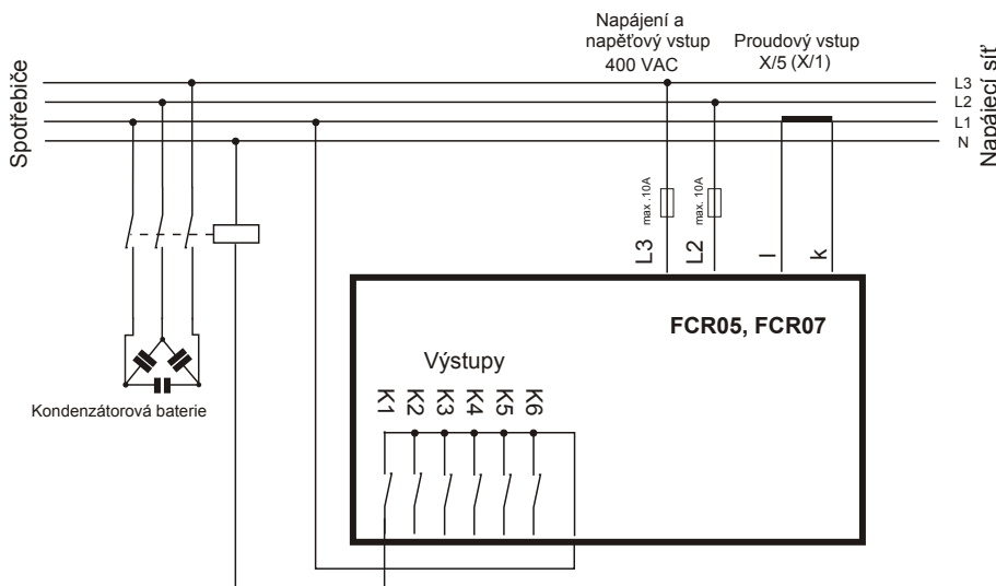
Obr. 3. Schéma připojení regulátoru pro stykačové stupně
